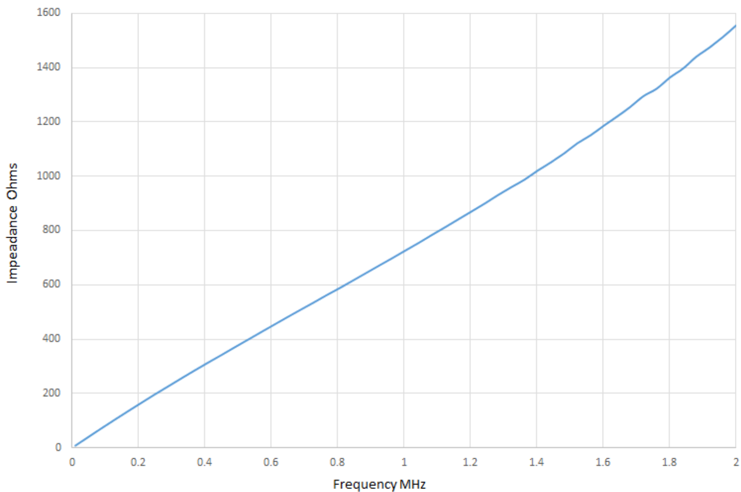
Rysunek 2 Ocena impedancji tłumienia baluna w paśmie od 10 kHz do 2 MHz
